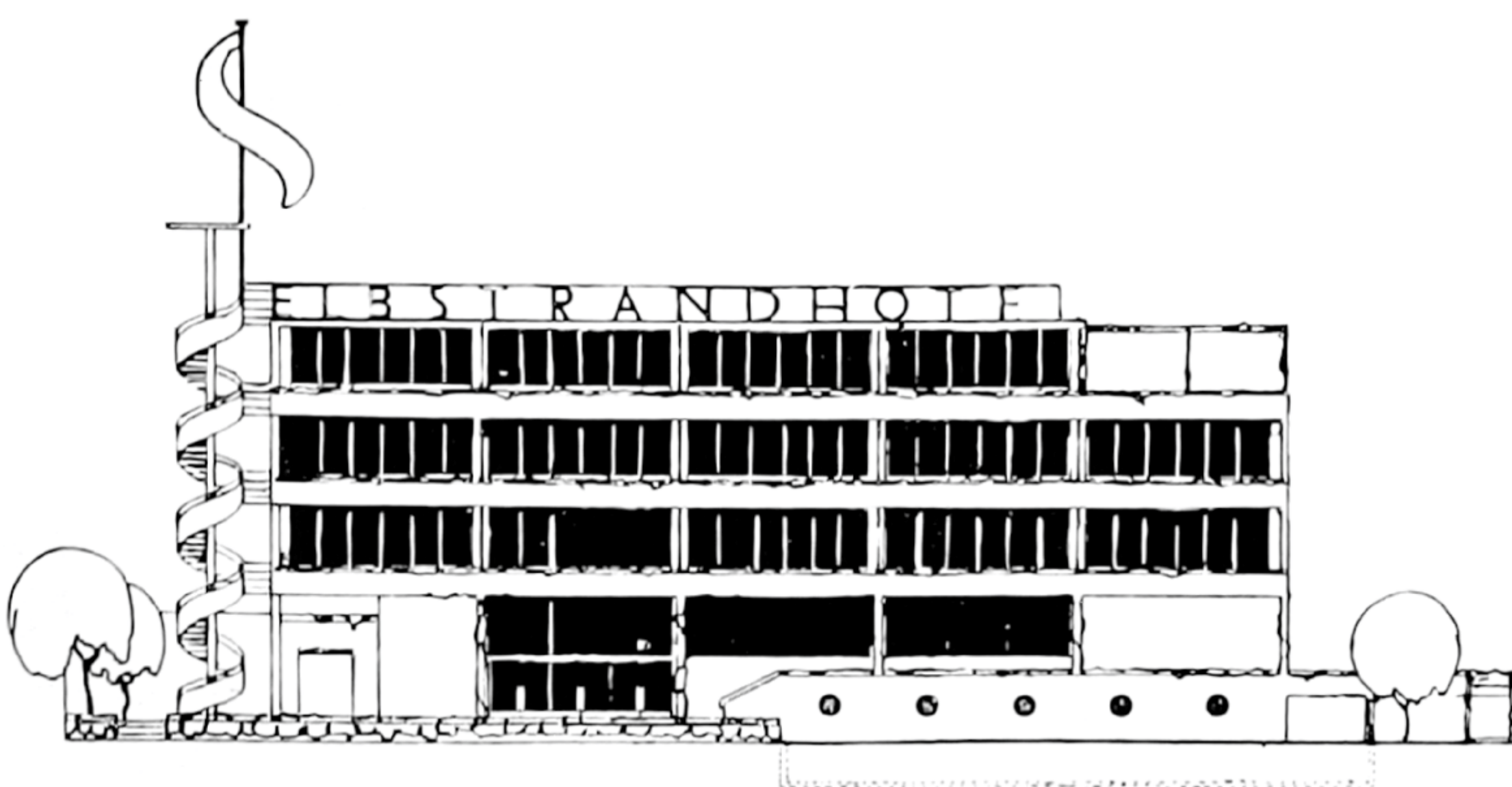
Obr. 2: Soutěžní návrh na hotel v Dolních Zálezlech (1929), nerealizovaný návrh společně s Wilhelmem Schütte, axonometrie, pohled do vstupní haly a vstupní průčelí
